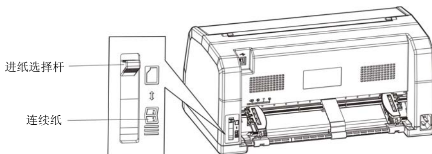
图 3-7 设定纸选择杆位置（连续纸）
